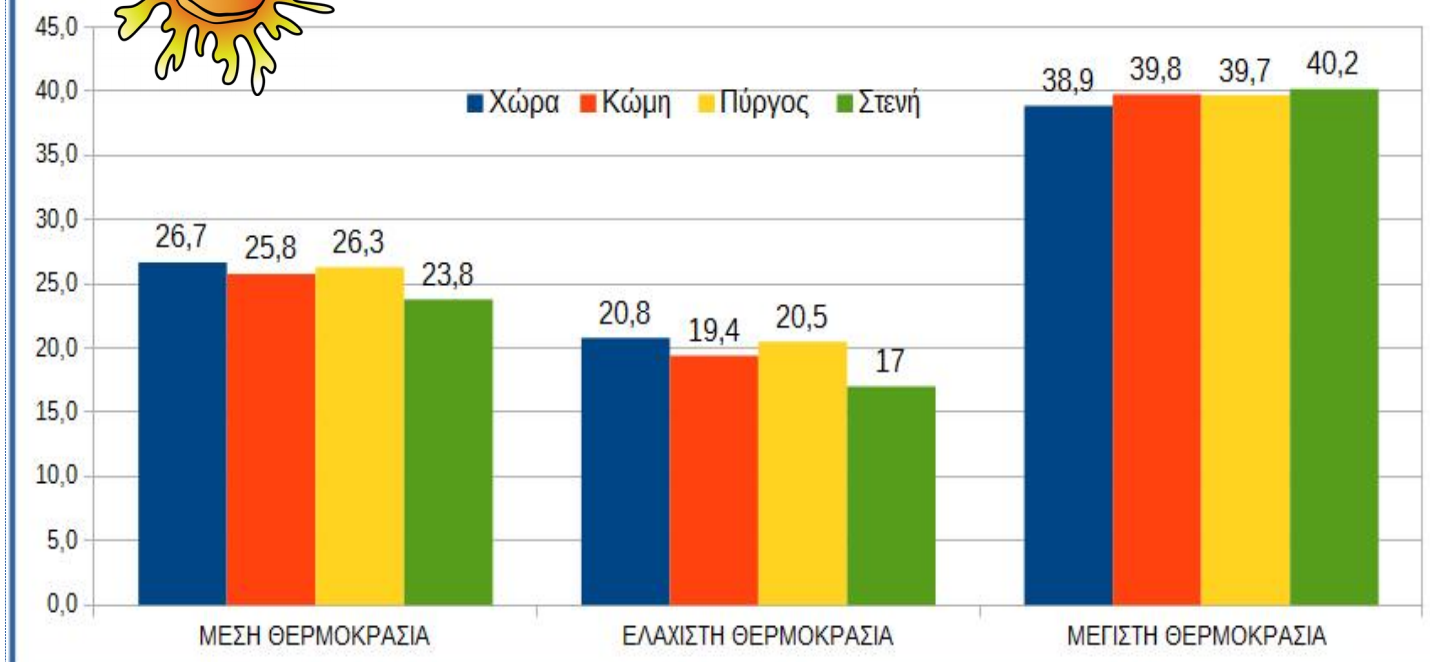
ΤΗΝΟΣ ΘΕΡΜΟΚΡΑΣΙΕΣ ΙΟΥΛΙΟΥ 2017
