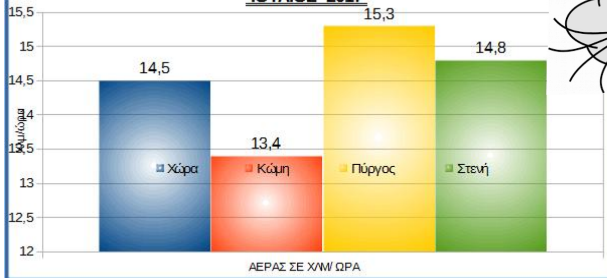
ΤΗΝΟΣ ΜΕΣΗ ΤΑΧΥΤΗΤΑ ΑΕΡΑ ΙΟΥΛΙΟΣ 2017
